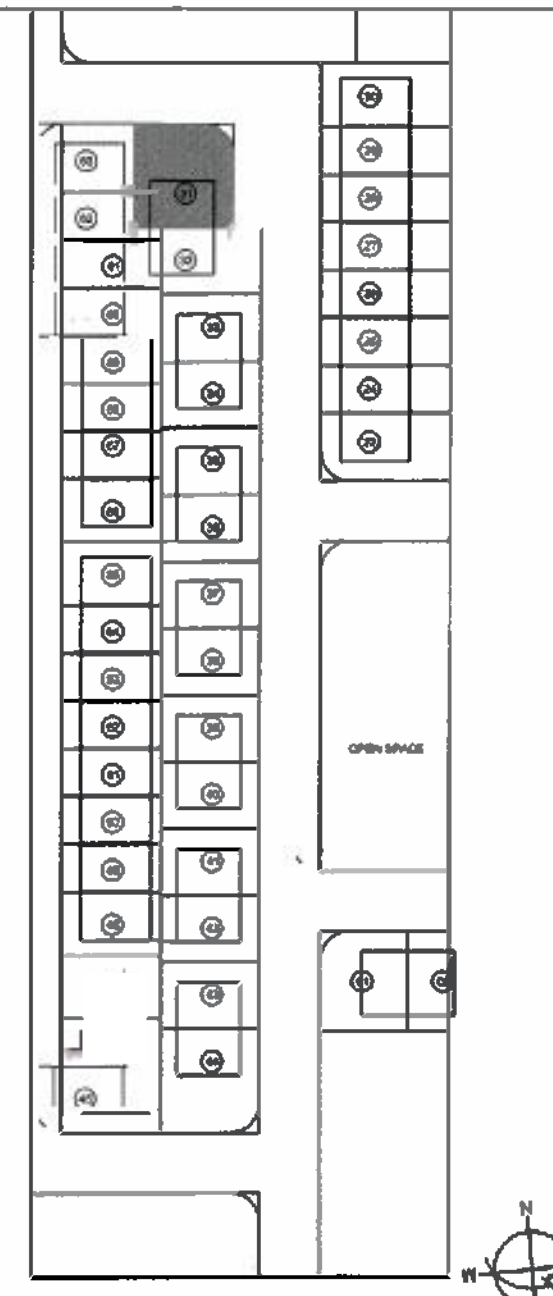
PLOT DEMARCATION PLAN SCALE - N.T.S.
