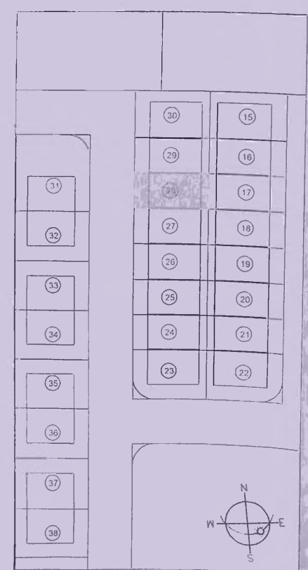
PLOT DEMARCATION PLAN SCALE - N.T.S.
