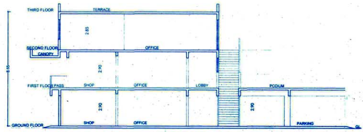
SECTION @ DD SCALE 1:100
