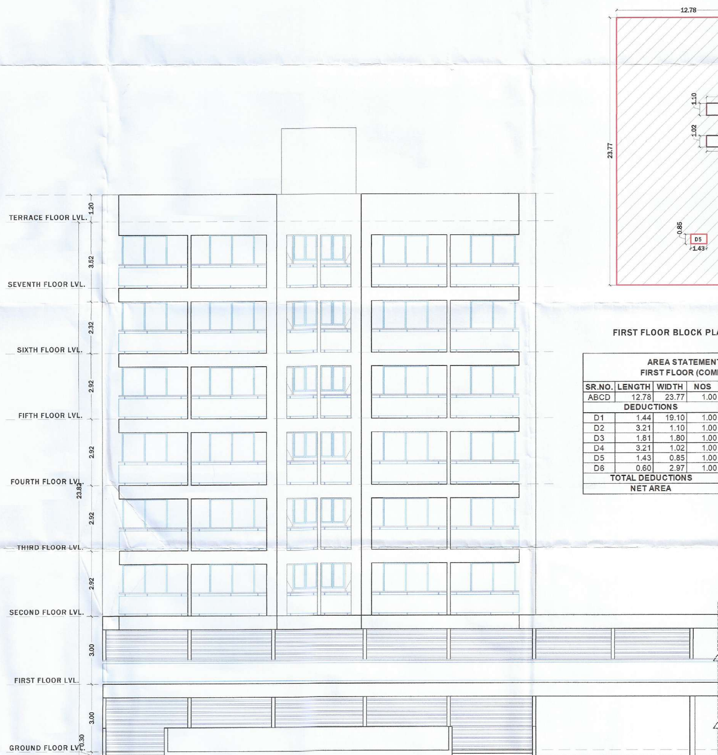
ELEVATION
