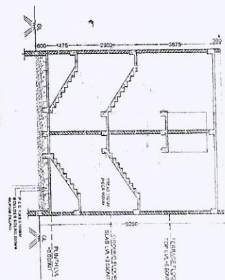
SECTION FF SCALE: 1:100
