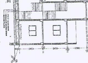
SECTION EE SCALE: 1:100
