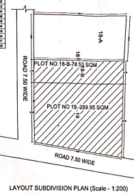
LAYOUT SUBDIVISION PLAN (Scale - 1:200)
