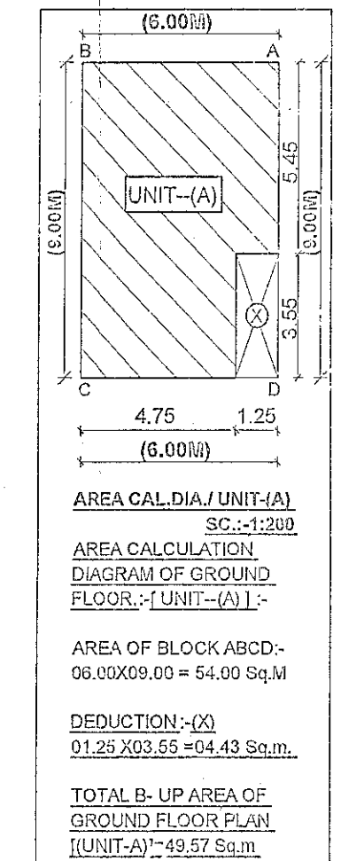
AREA CALC. DIA. / UNIT-(A) SC:-1:200
